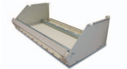
Dimensions du présentoir 100 × 51 × 27 cm
